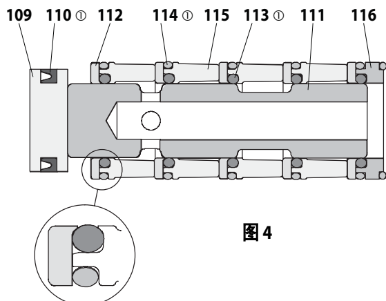
主阀门剖视图
